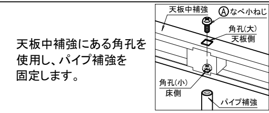
天板中補強とパイプ補強の固定方法と注意点
